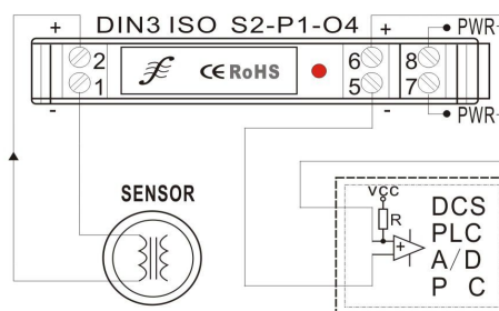
DIN3 SY S-P-O集电极开路输出接线图
